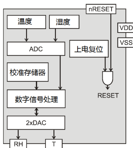
图 2 GXHT31 功能原理框图
